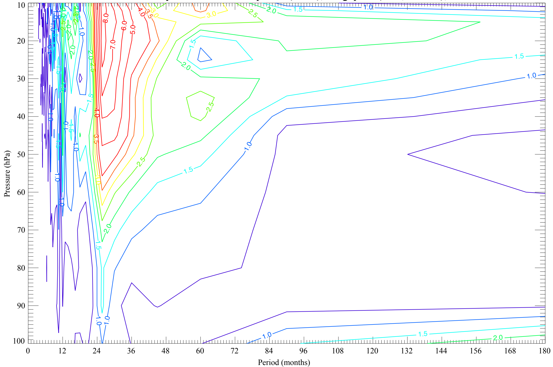
NCEP Reanalysis Wind Power Spectra ( \text{m}\cdot\text{s}^{-1} ), Singapore ( 1^\circ\text{ N} , 104^\circ\text{ E} ), 1948–2004
